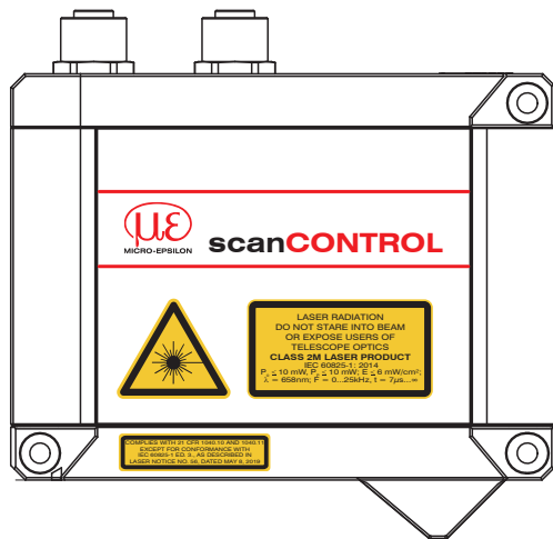
Sensor with laser labels, LLT30xx-25, LLT30xx-50, LLT30xx-100, LLT30xx-200
