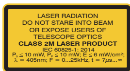
Laser warning sign and laser label LLT30xx-25/BL, 30xx-50/BL, 30xx-100/BL
